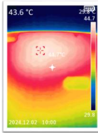
อุณหภูมิ Inverter NO.5 44.7 °C 18SNPB-WIV0
