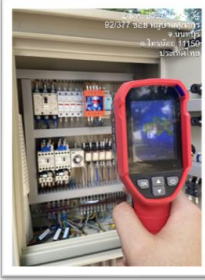
อุณหภูมิความร้อน 41.9 °C
