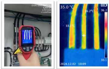
ตรวจสอบความร้อนสาย MCCB 36.2 °C
