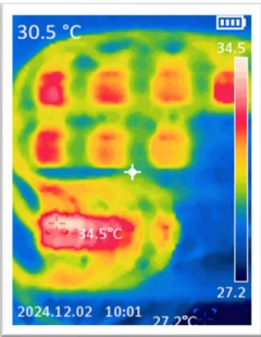
อุณหภูมิ 34.5 °C 18SNPB-WDC01
