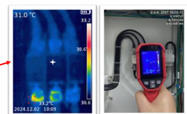
ตรวจสอบความร้อนสายไฟฟ้า MCCB 33.2 °C
