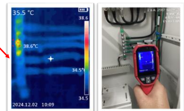
ตรวจสอบความร้อนสายกราฟต์ MCCB 38.6 °C
