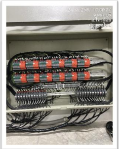
ตรวจสอบสภาพและความพร้อมของอุปกรณ์ภายใน Dc Panel Box No.5 18SNPB-WDC01
